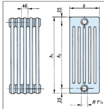
Altı sıra modelinde çelik boru radyatörlerinin ölçüleri
