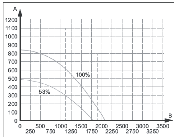
A: Basma yüksekliği (mbar) B: Sirkülasyon miktarı (l/h)
