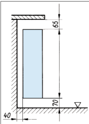
Radyatör boşluğuna montaj
