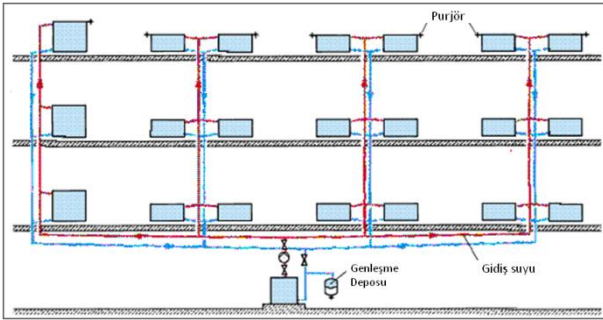
Alttan dağıtım çift borulu bir kaloriferin boru döşeme şeması
