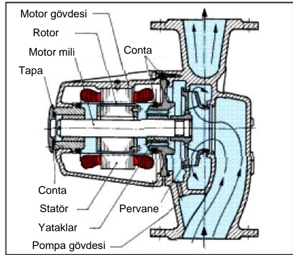
Flanş bağlantılı ıslak kovanlı pompa
