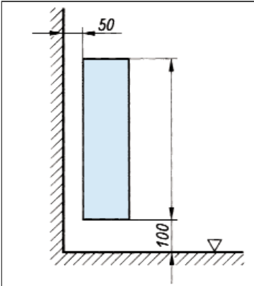
Serbest olarak monte edilen radyatör
