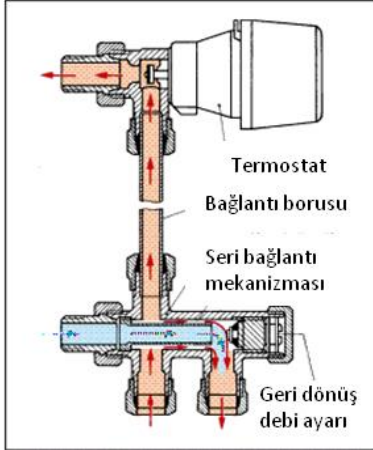
Termostatik vanalı seri bağlantılı mekanizma
