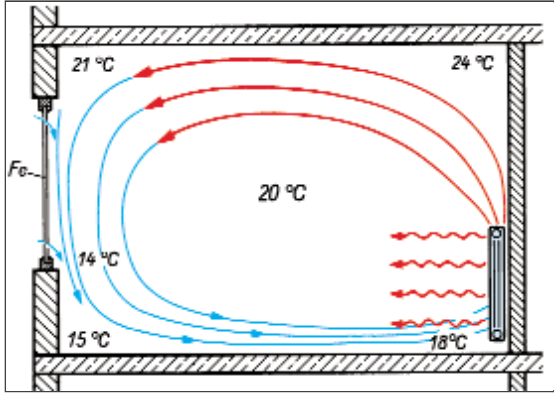
Dengesiz oda sıcaklığındaki iç duvar radyatör düzeni
