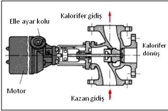
Motorlu üç yollu vana
