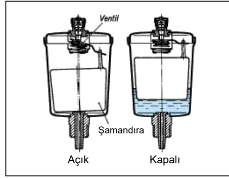
Otomatik hava purjörünün çalışma şekli
