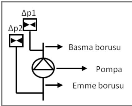
Pompa basıncının ölçümü
