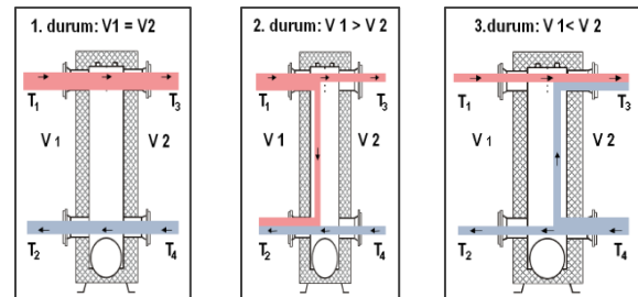
Isıtma cihazı ve tesisat debisine göre hidrolik karıştırıcı çalışma durumları
